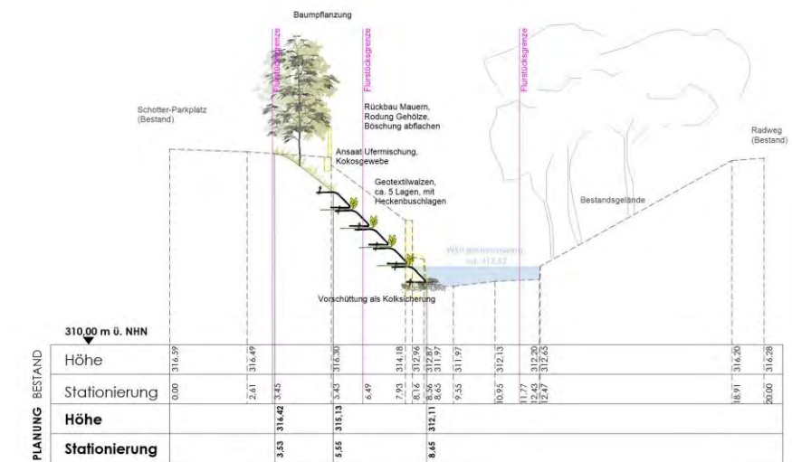
Profil 1 M 1:100
