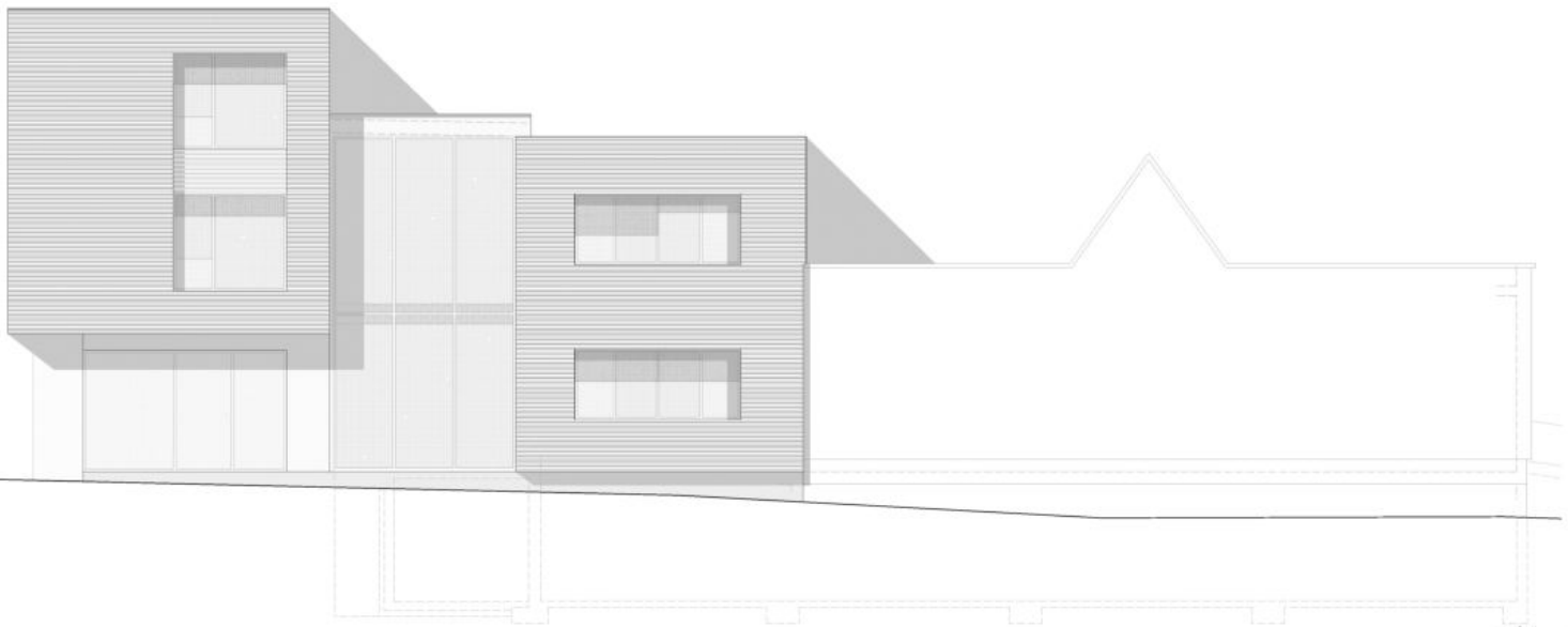
ansicht nord
