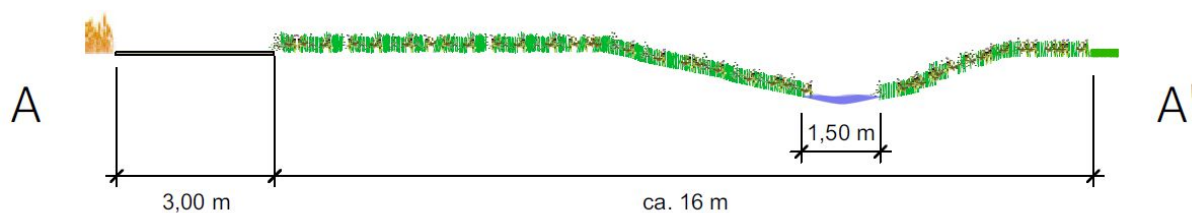
Abb. 3: Querschnitt durch den geplanten Bachlauf (siehe auch Planskizze im Anhang)
