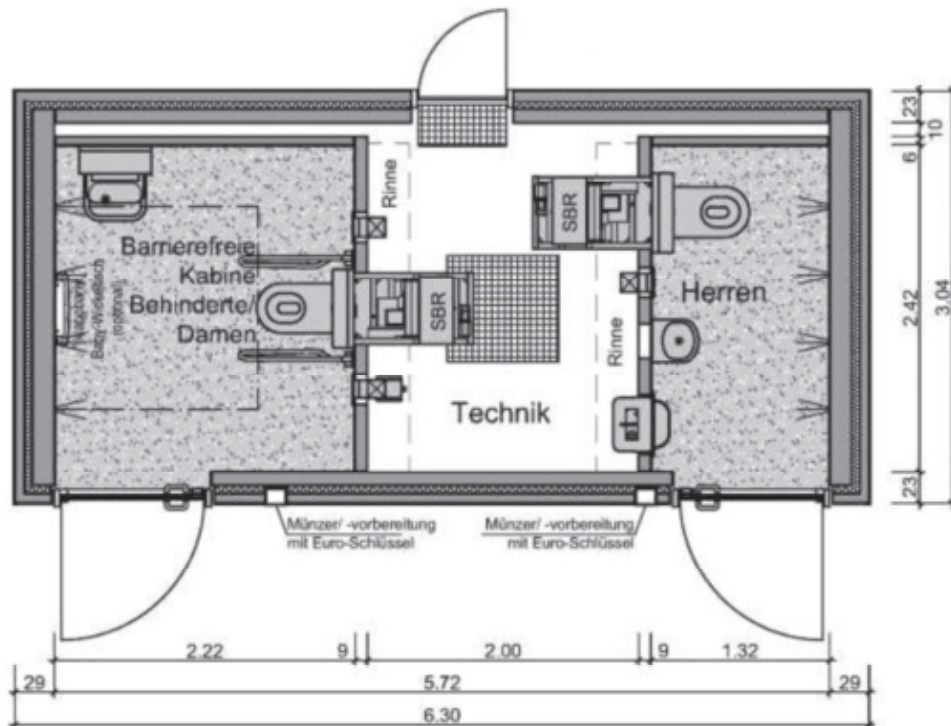
Beispiel für Zweiraum-WC, davon ein Raum behindertengerecht
