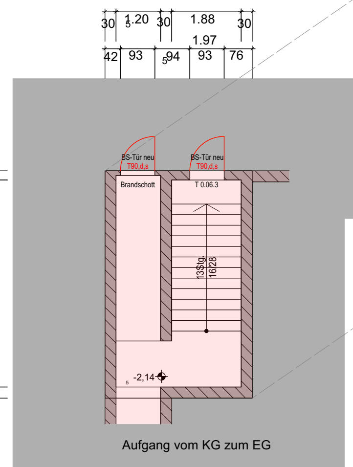
GRUNDRISS UG
