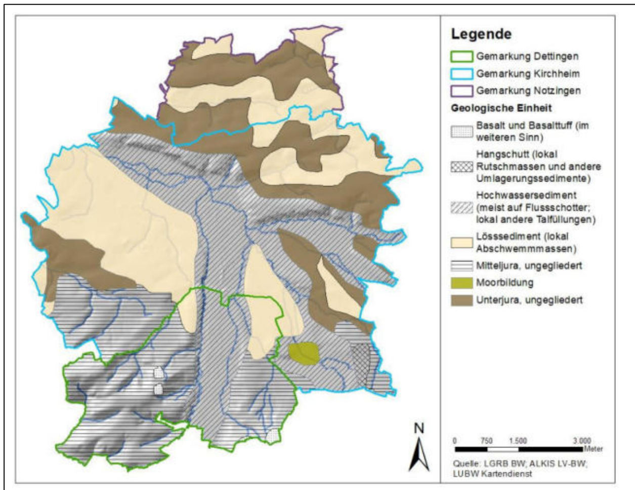
Abbildung 2: Geologische Einheiten im Planungsgebiet
