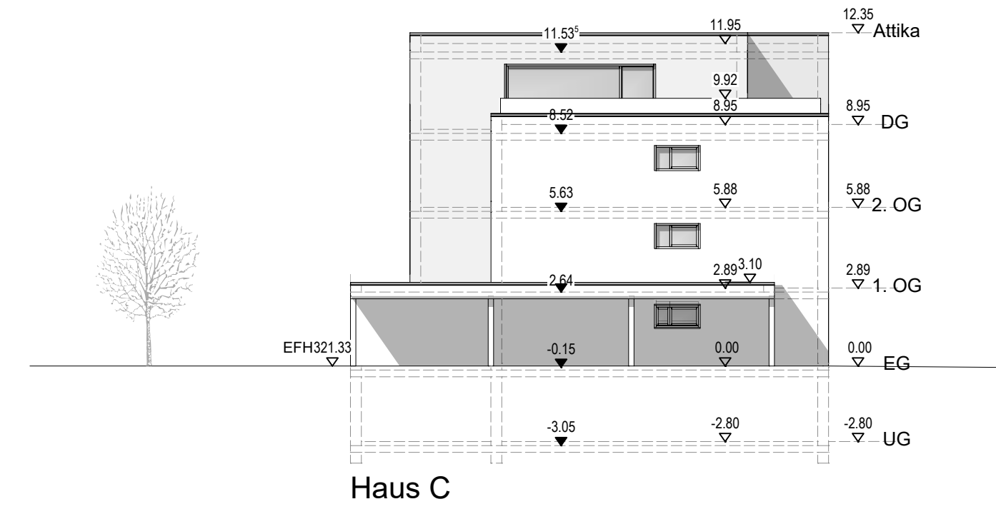
Ansicht Nord
