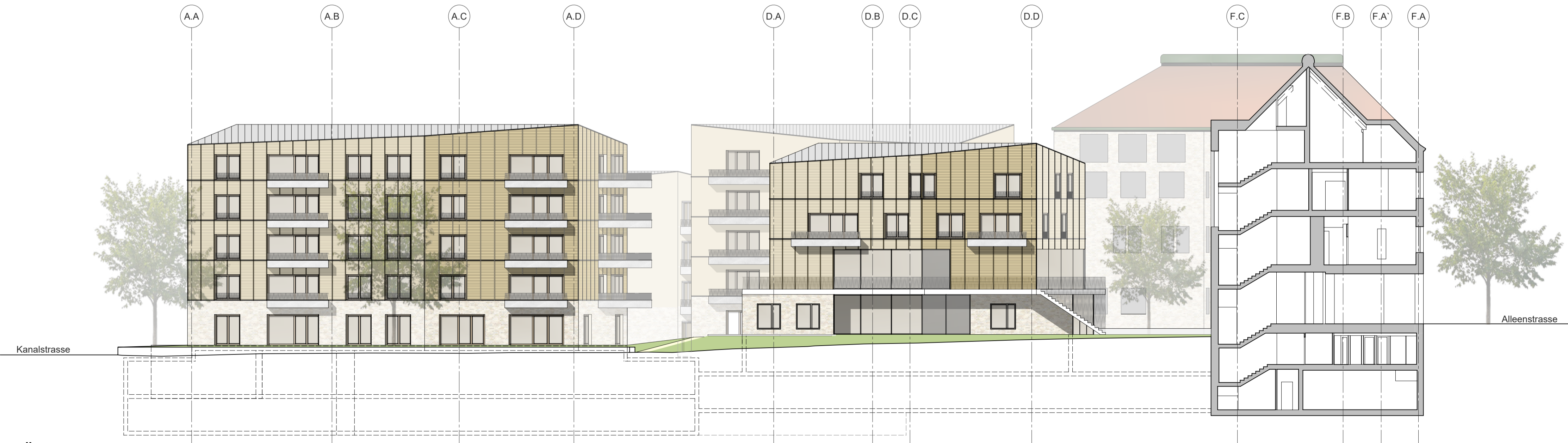
ANSICHT SÜD-WEST
